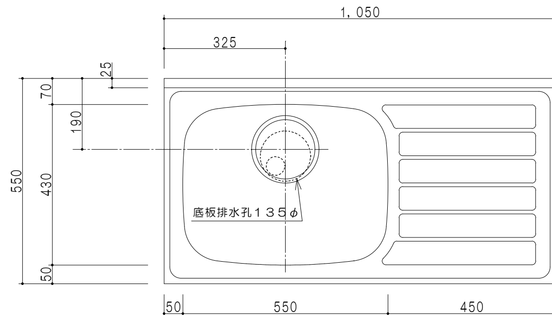
平面図
