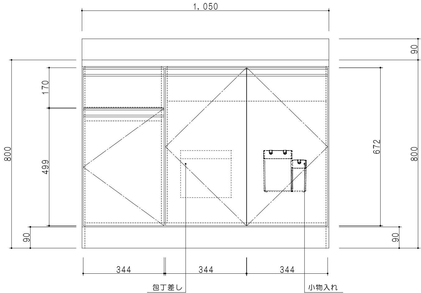
立面図
