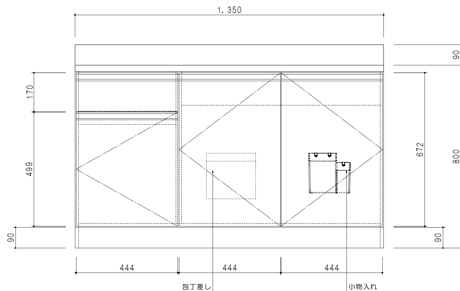
立面图
