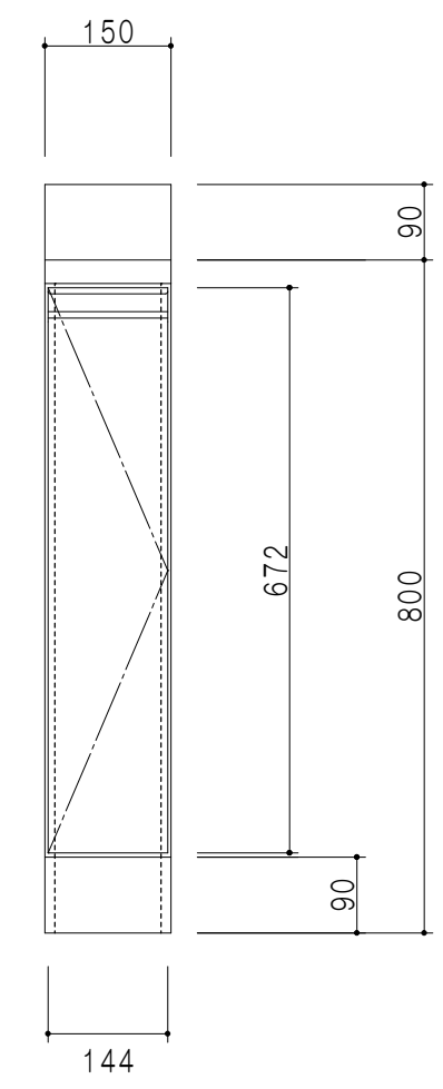
立面図
