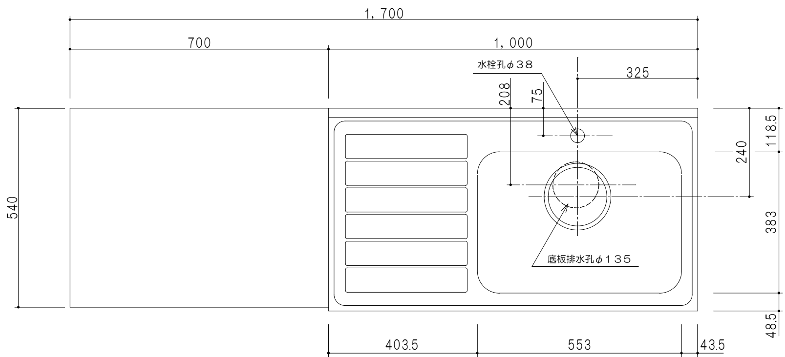
平面図
