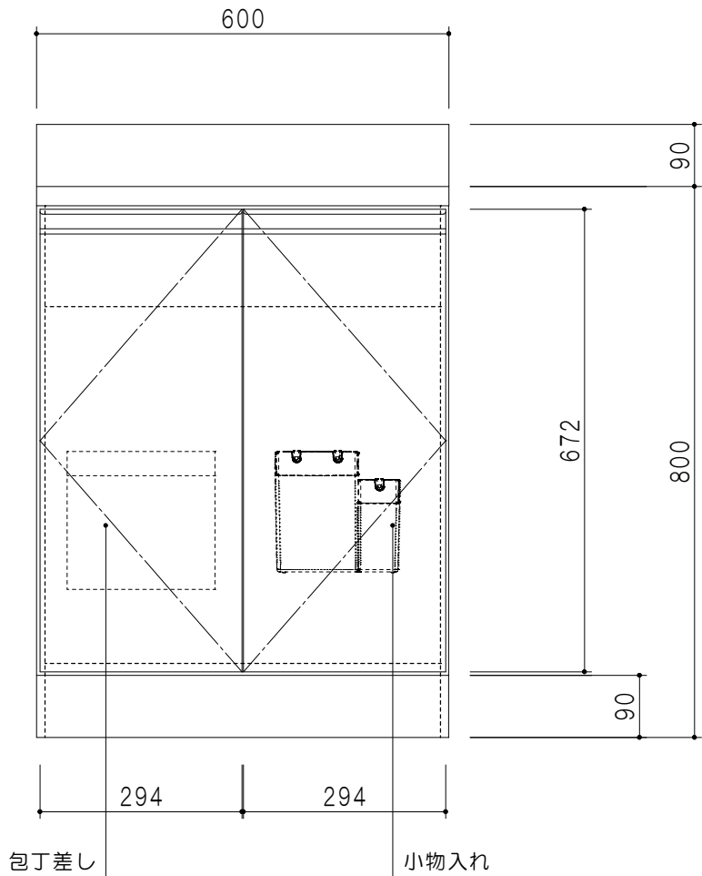
立面図
