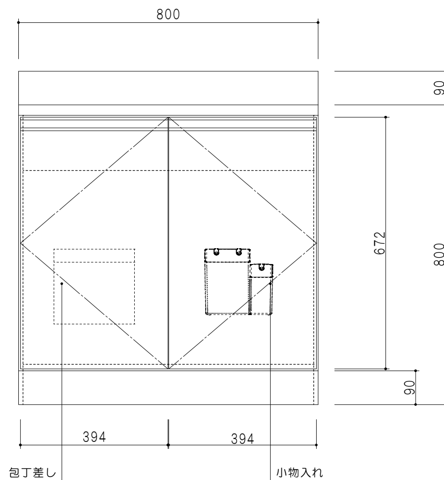
立面图
