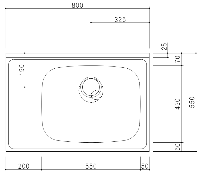
平面图
