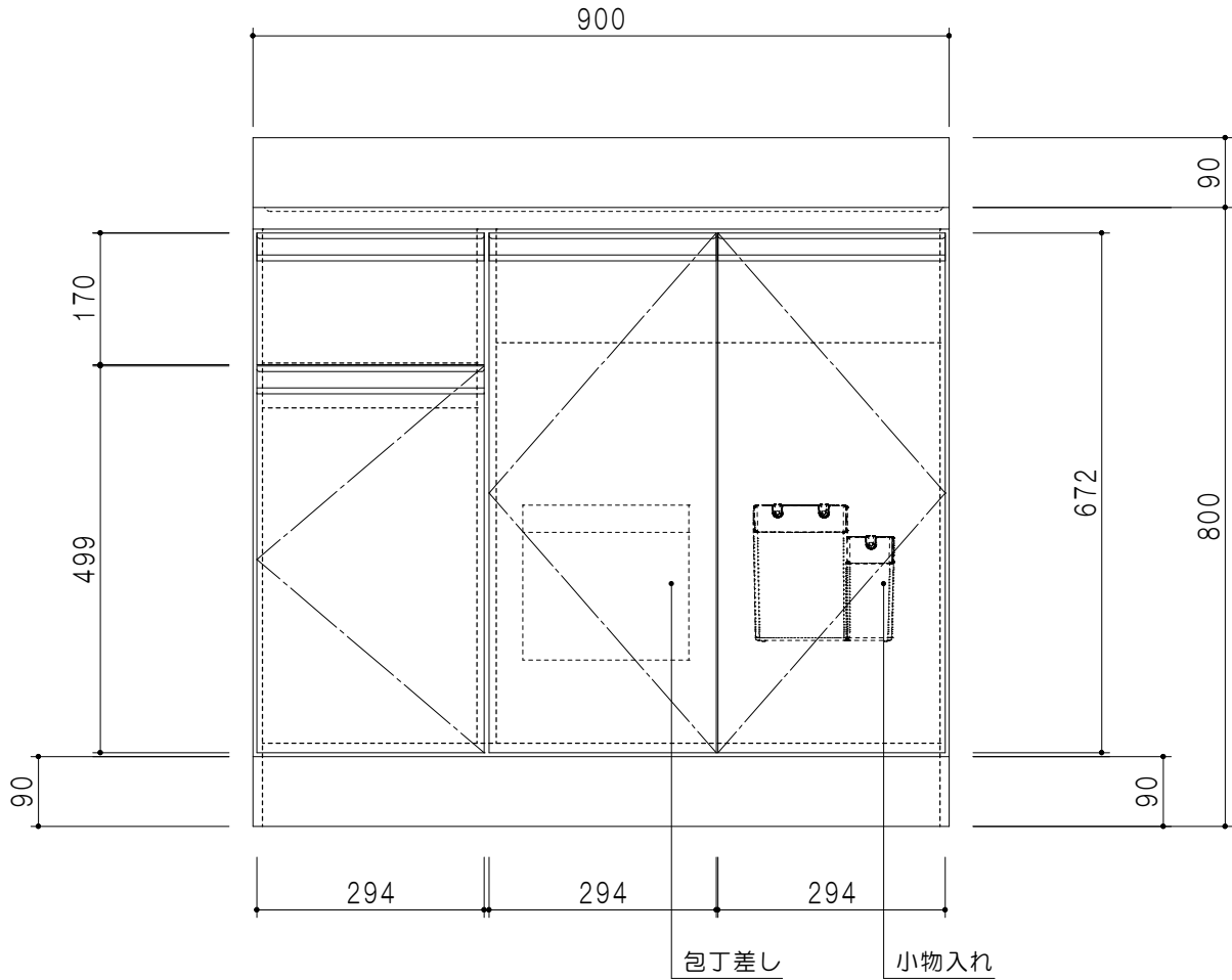
立面図
