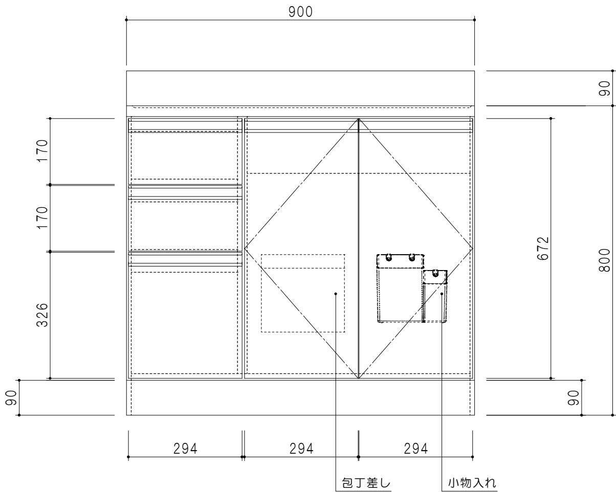
立面図
