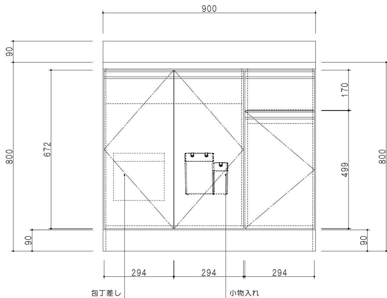
立面図
