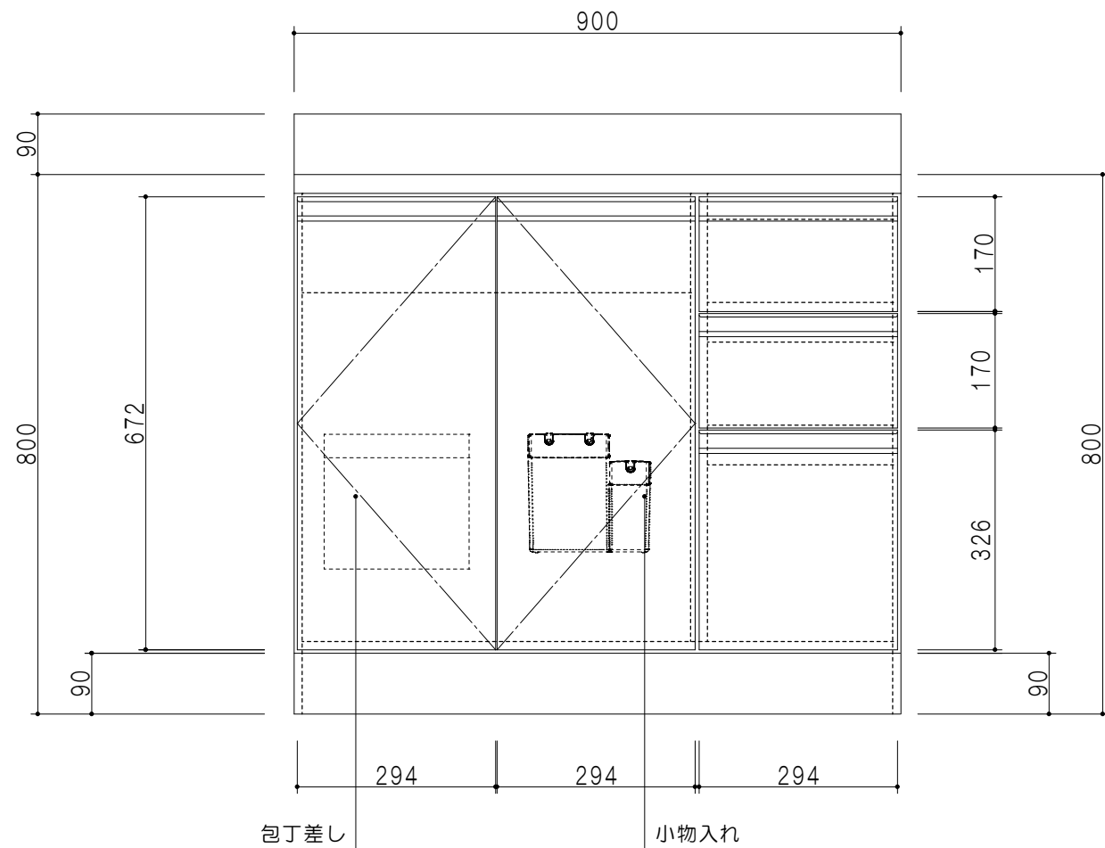
立面図
