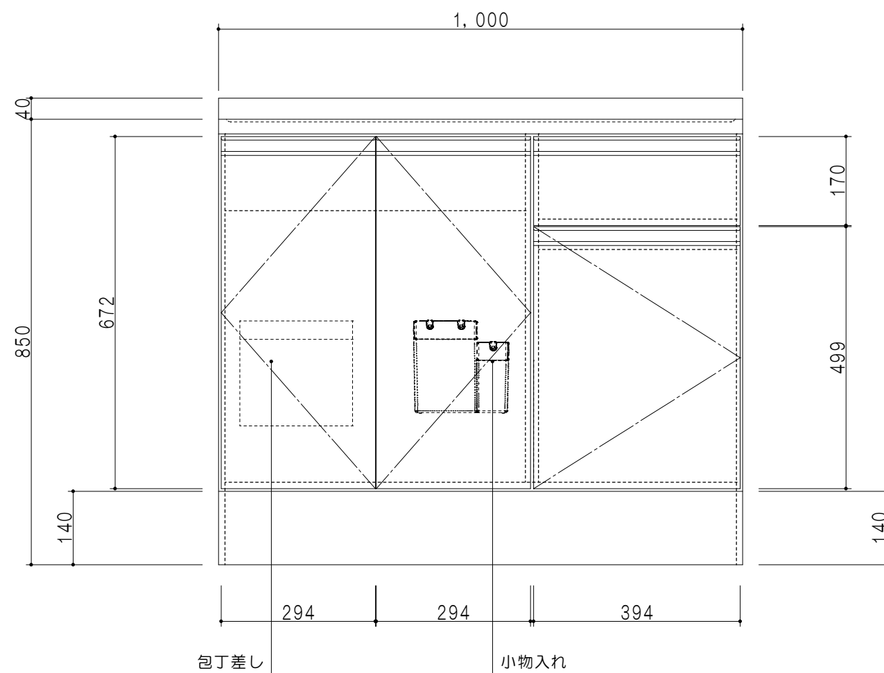
立面图
