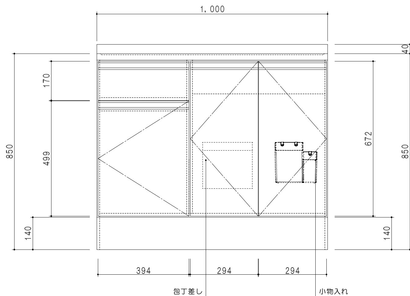
立面图
