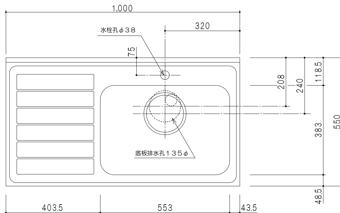
平面图
