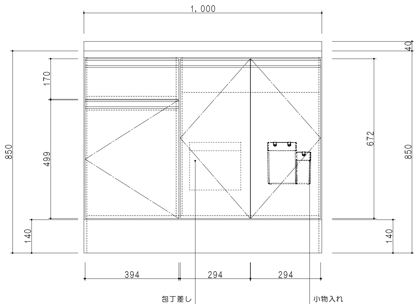
立面図
