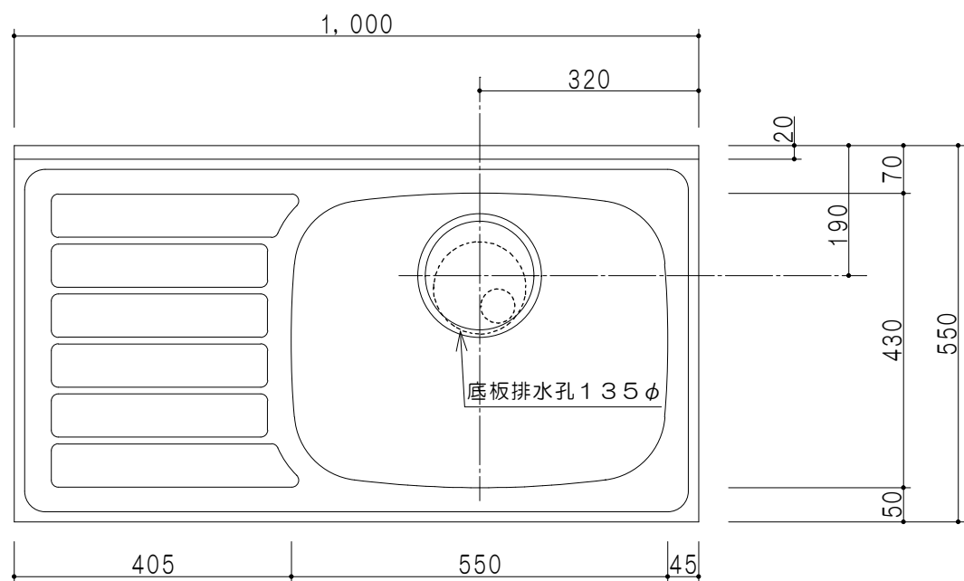
平面図
