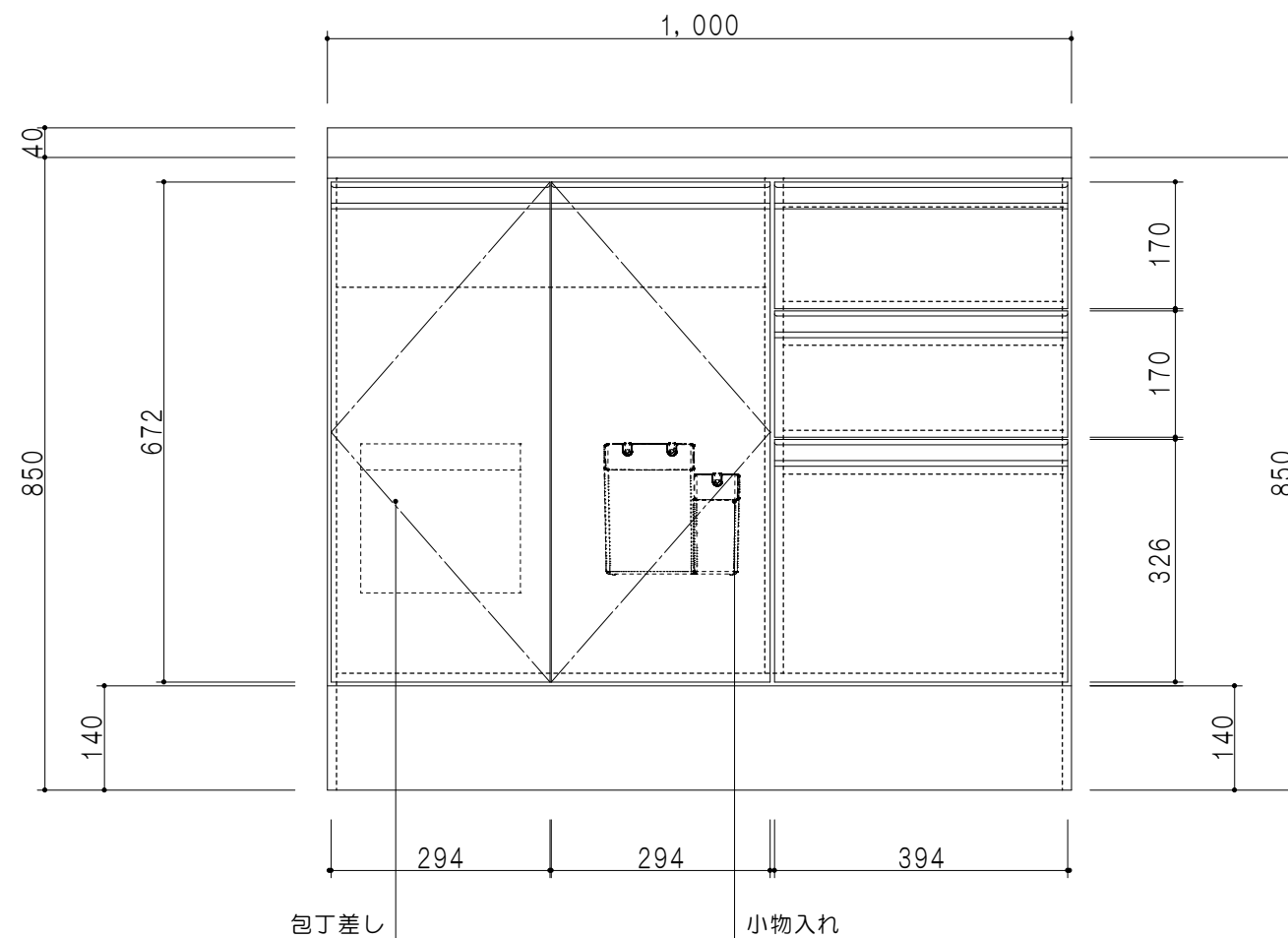
立面図
