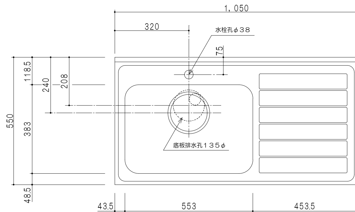
平面图
