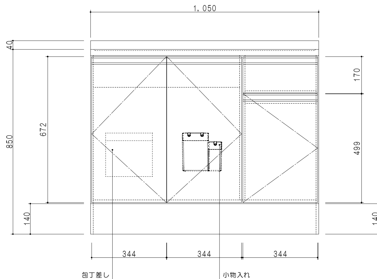
立面图
