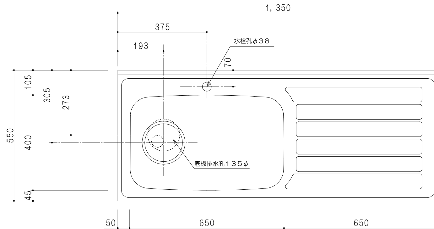
平面图
