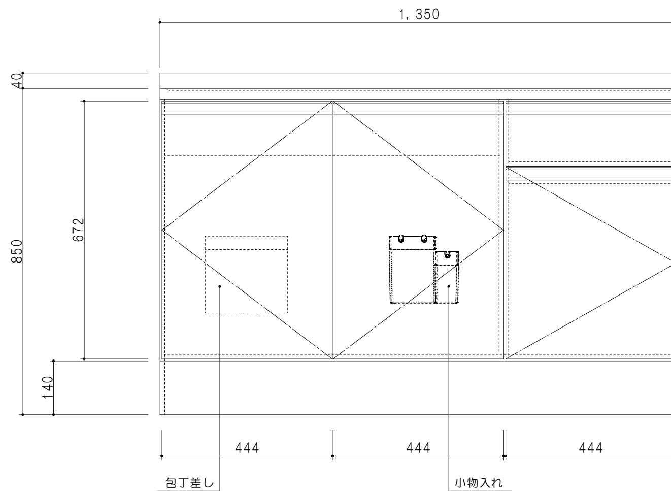
立面图
