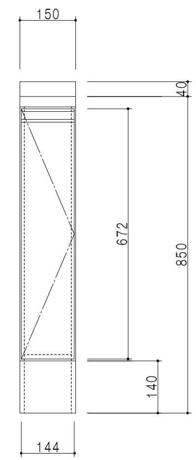
立面図
