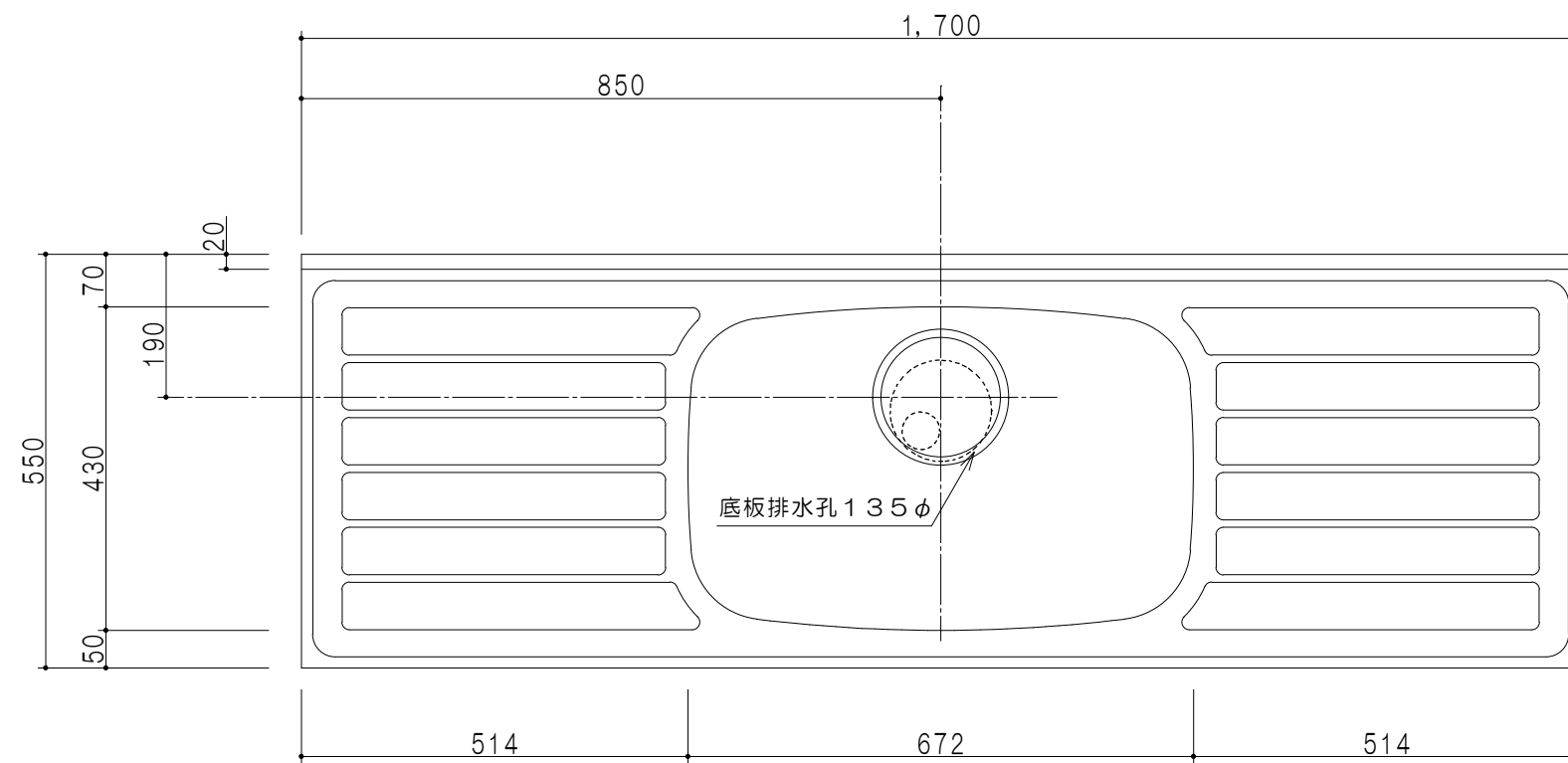
平面图
