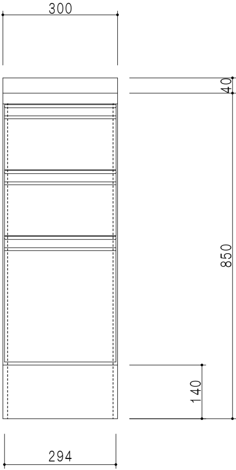
立面図
