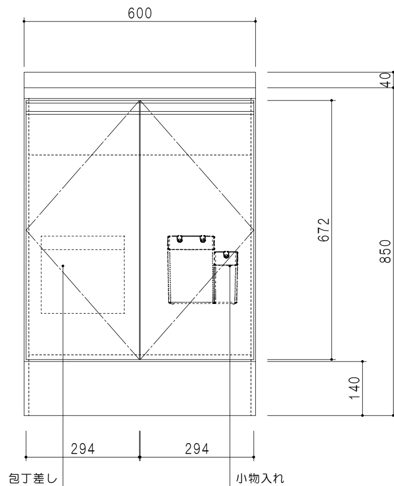
立面图
