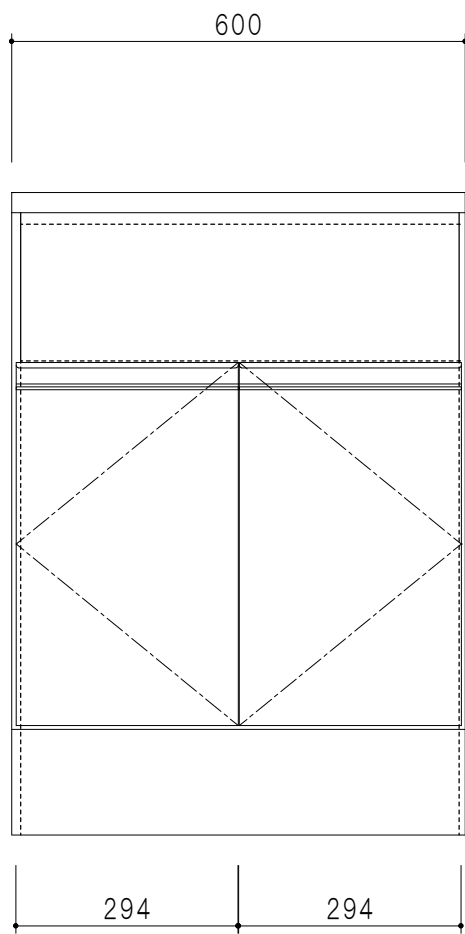
立面図
