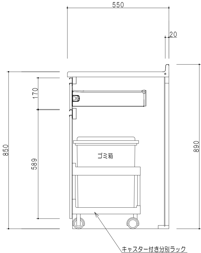
断面図
