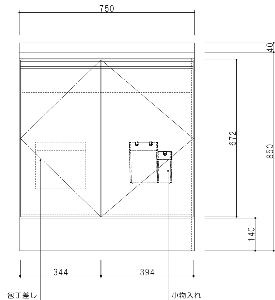
立面図
