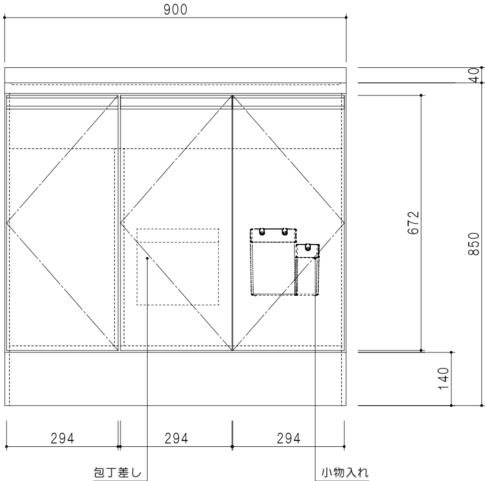
立面図
