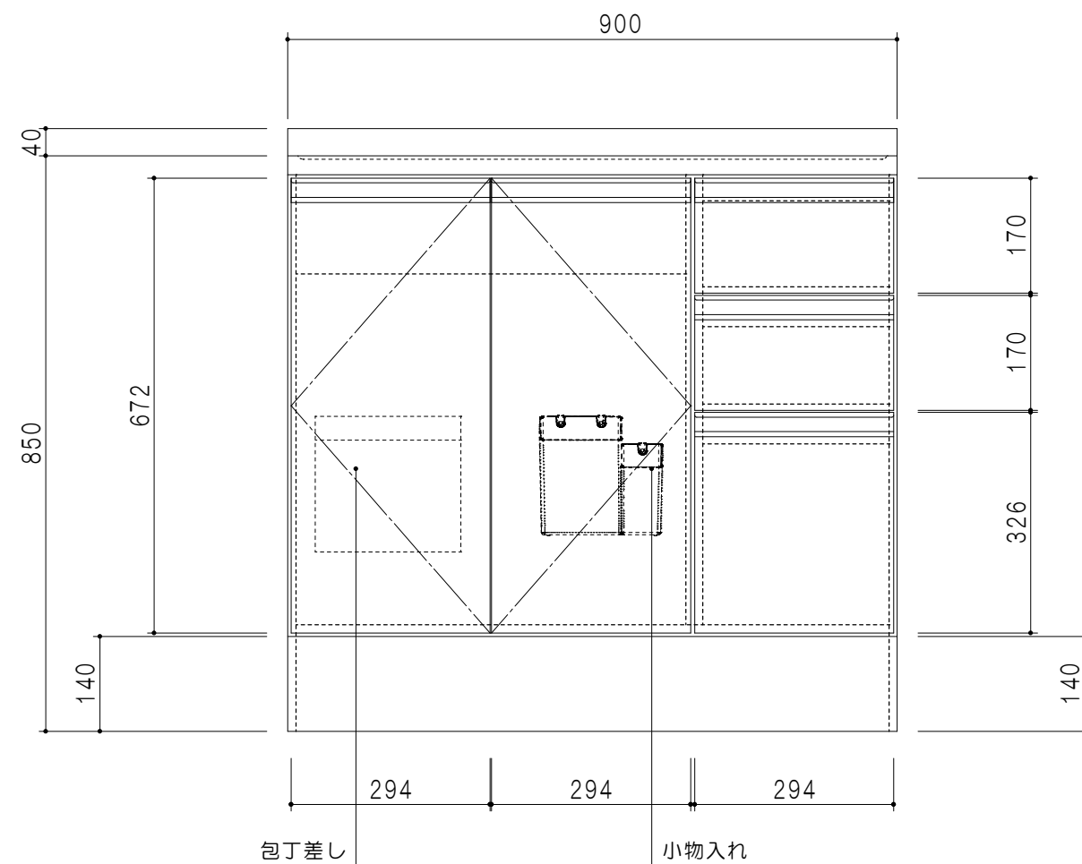
立面図
