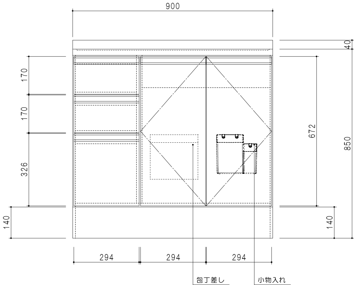
立面図
