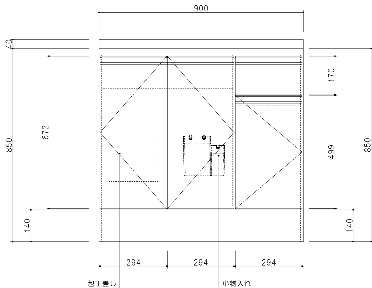
立面図
