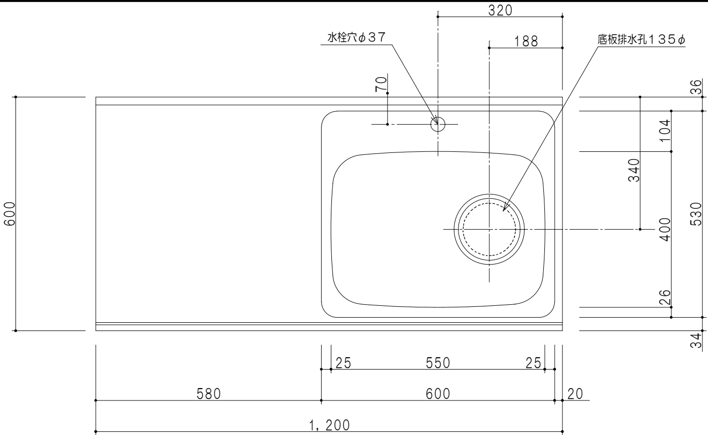
平面図
