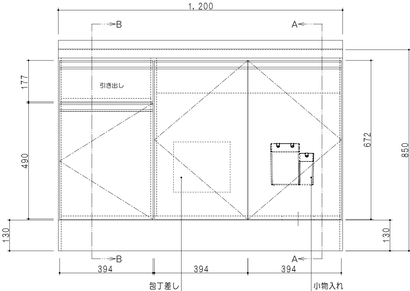
立面図
