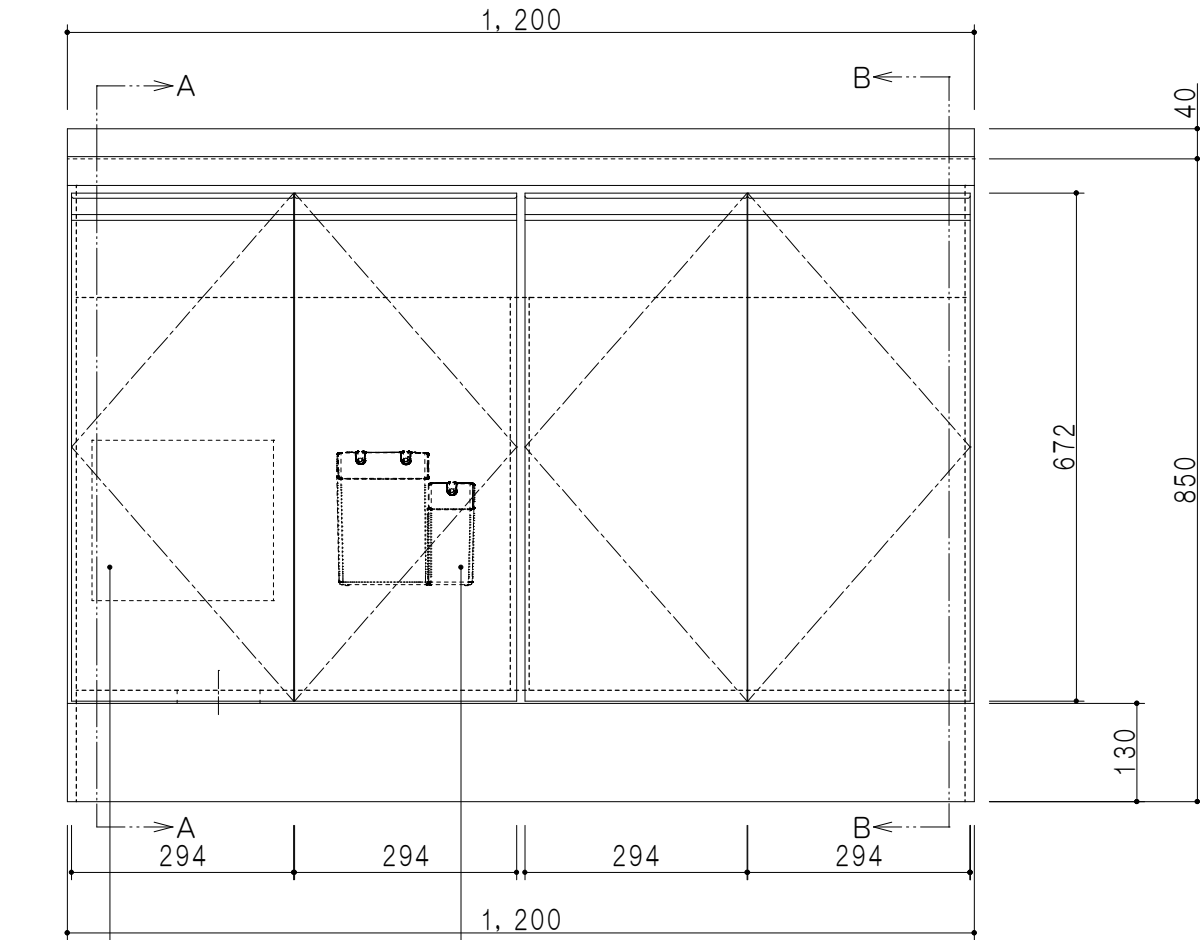
立面図
