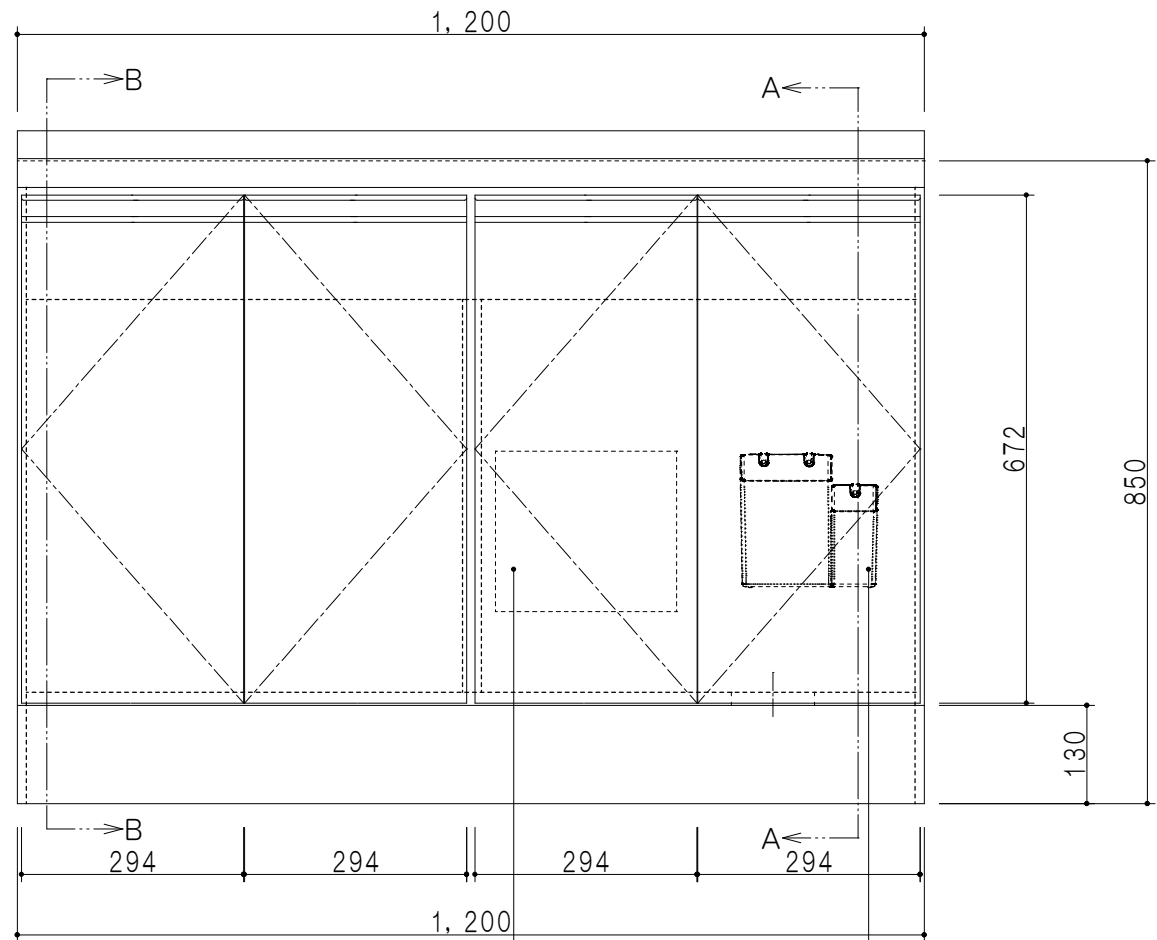
立面図
