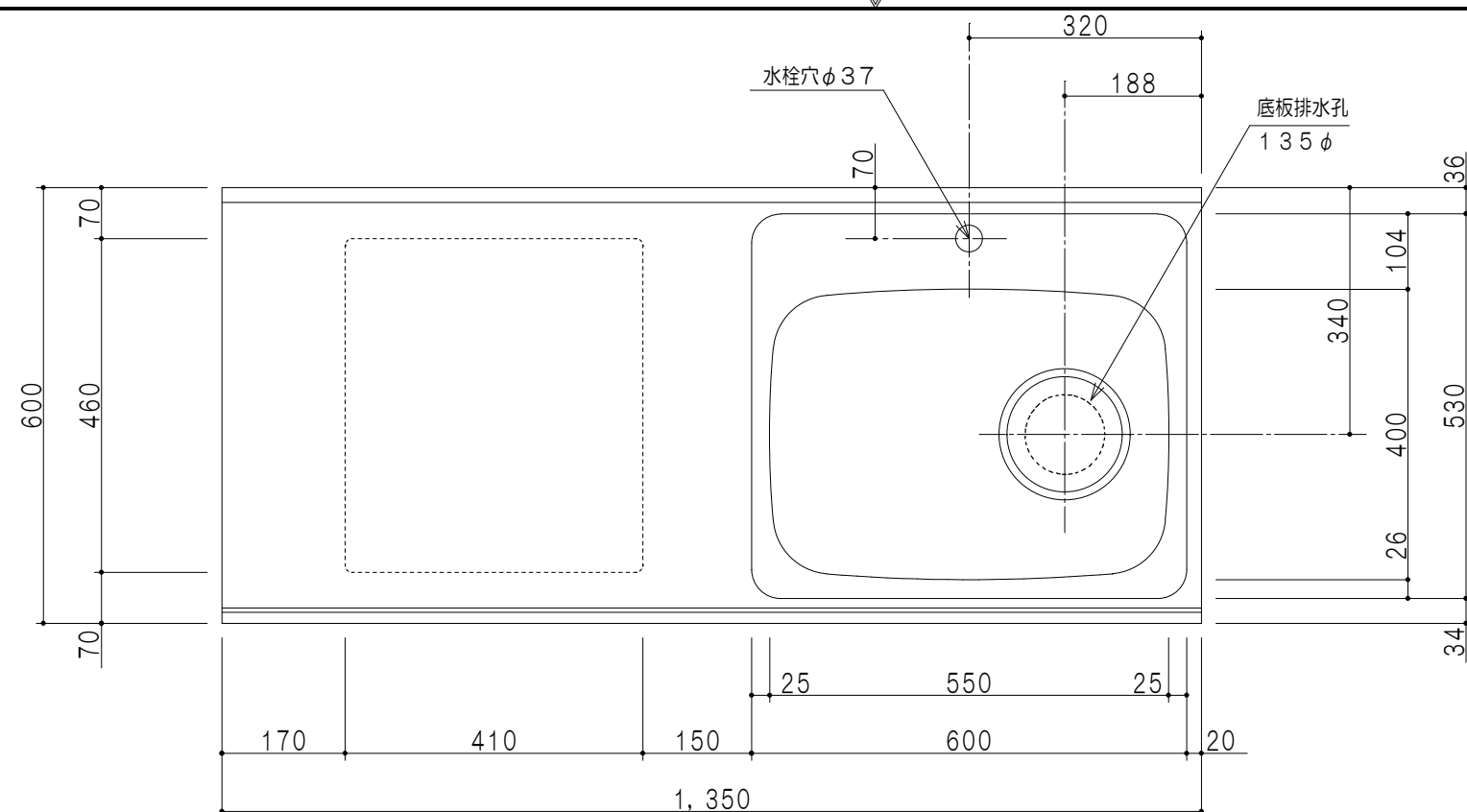
平面图
