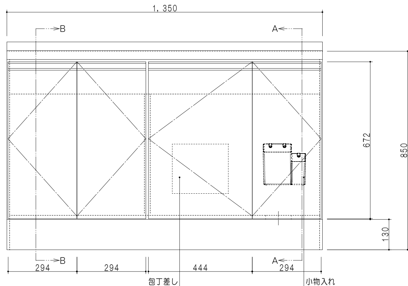
立面图
