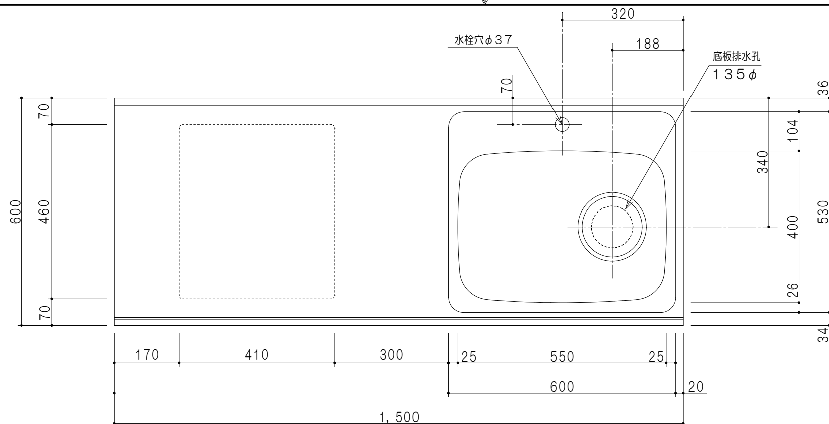
平面图
