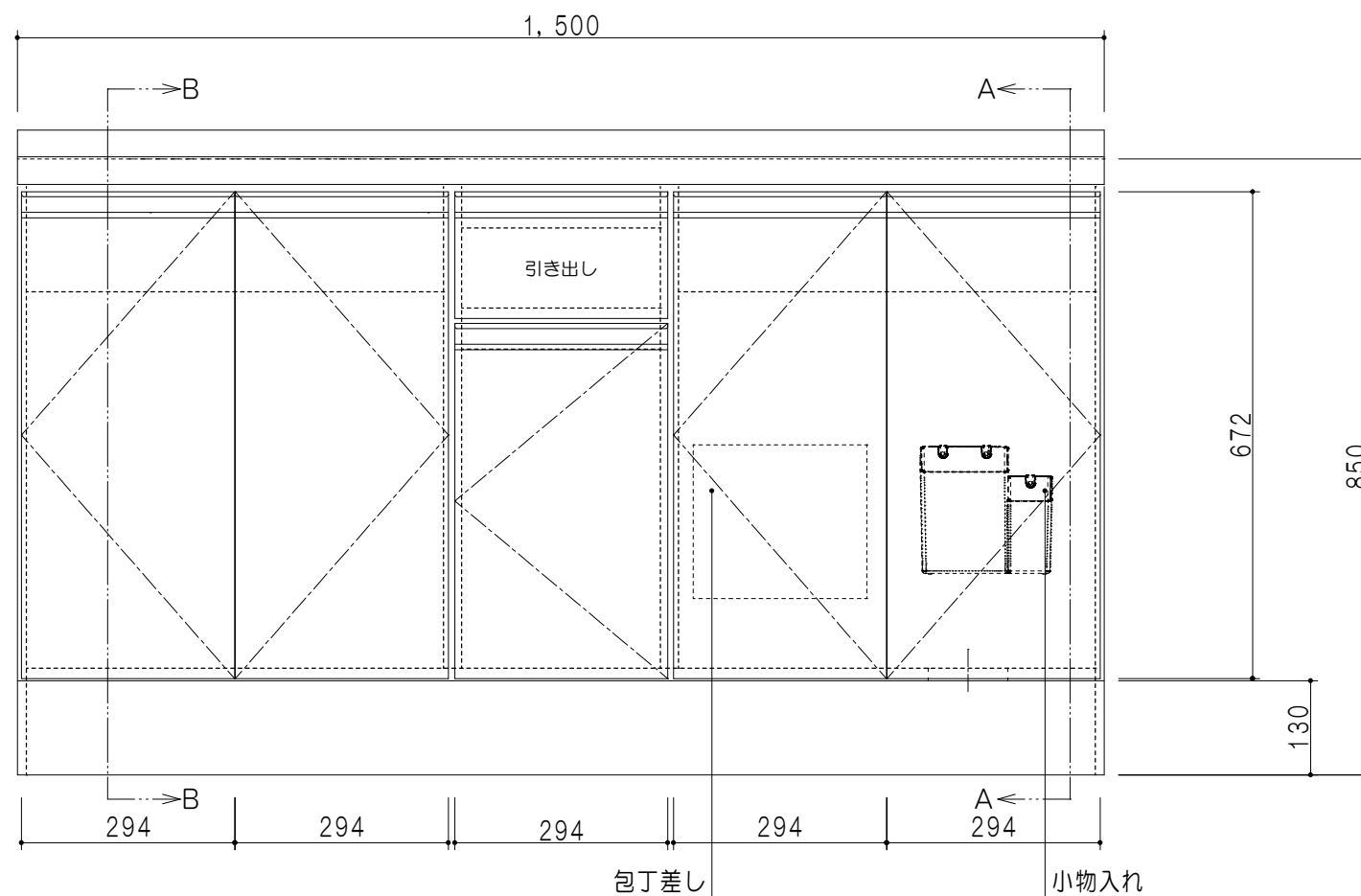
立面图
