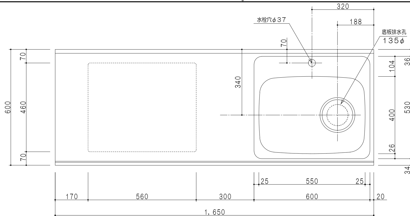
平面图
