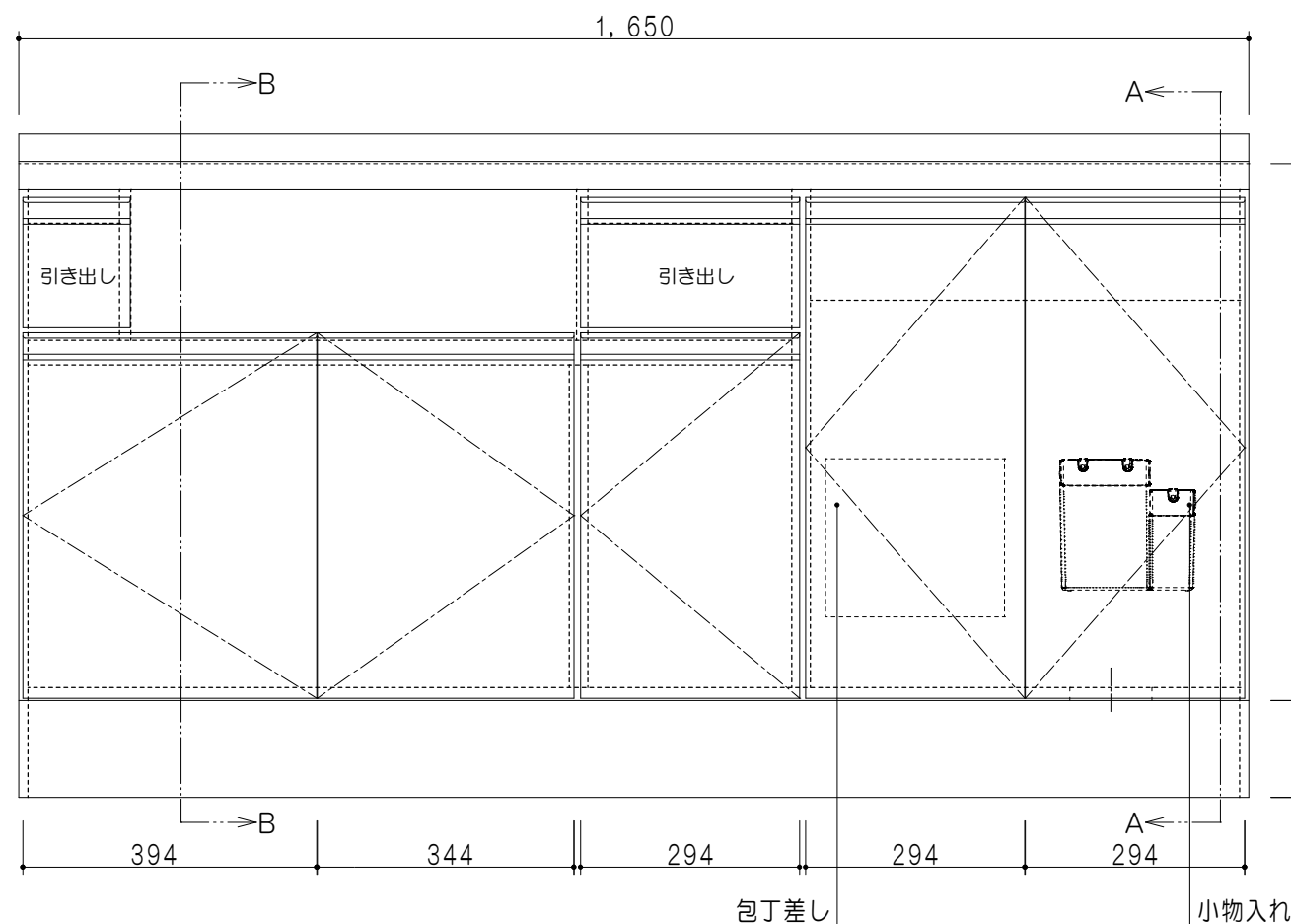
立面图
