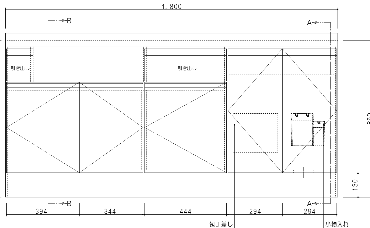
立面图
