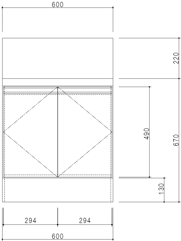
立面図
