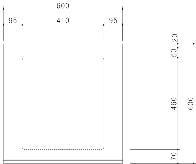
平面図
