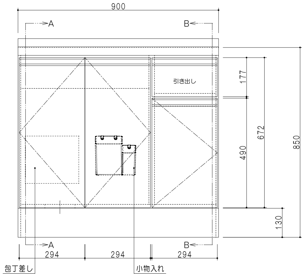
立面図
