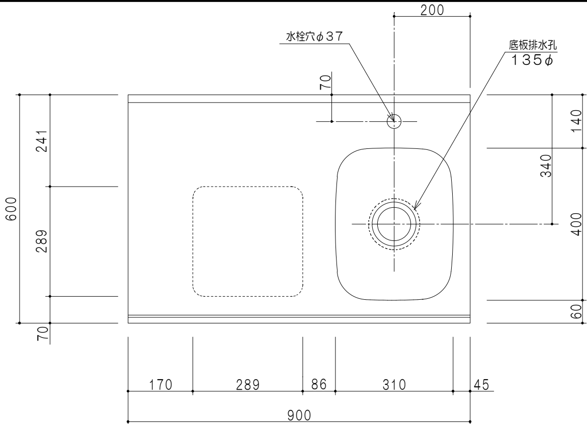
平面図
