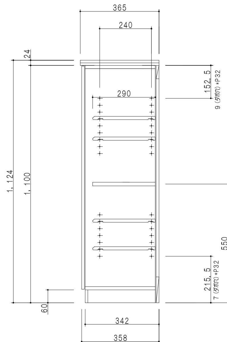
断面図
