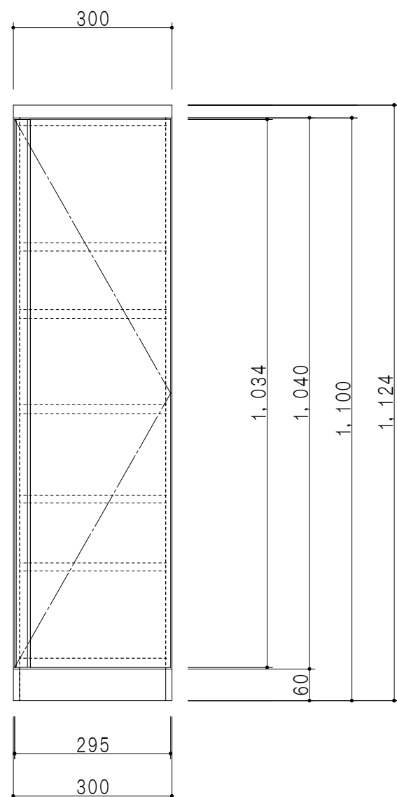
立面图
