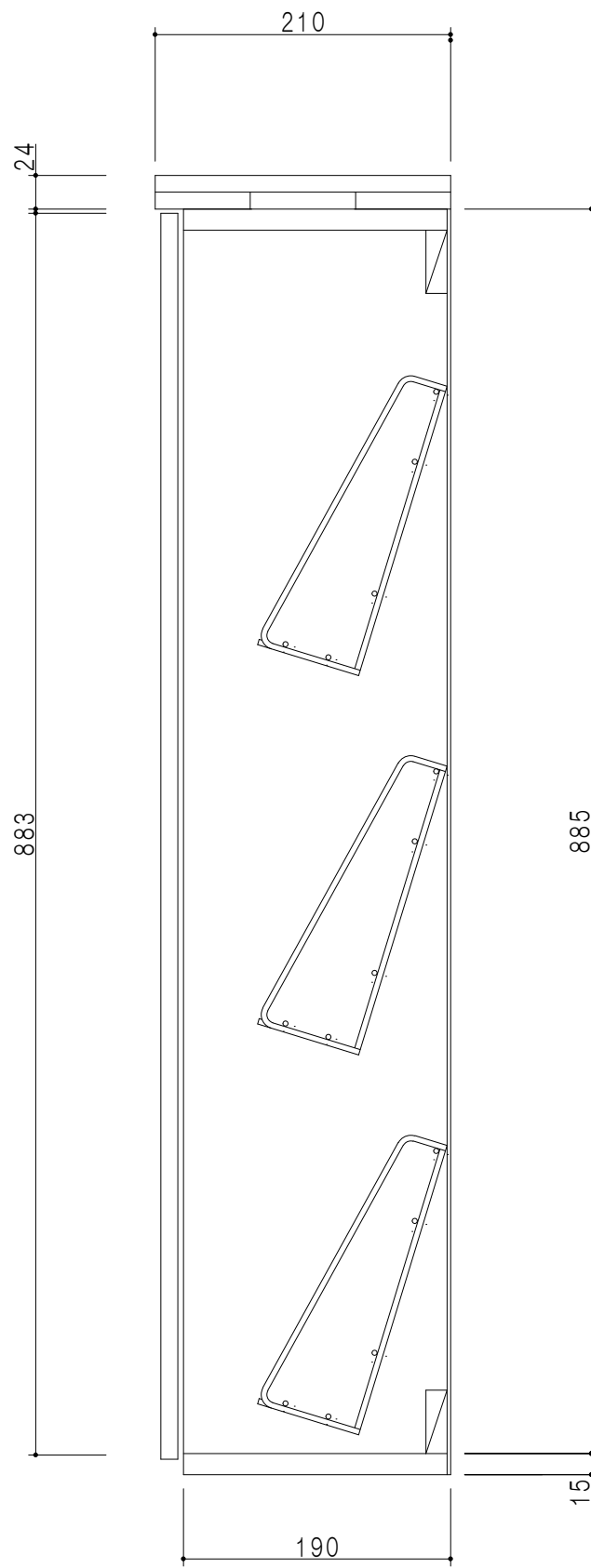
断面図
