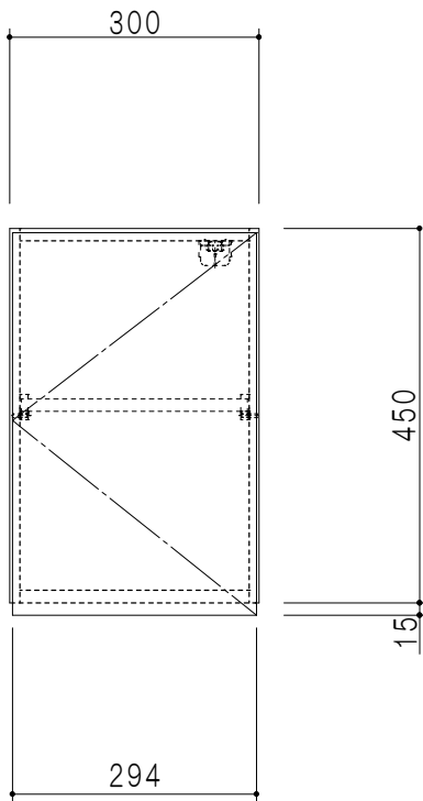
立面図
