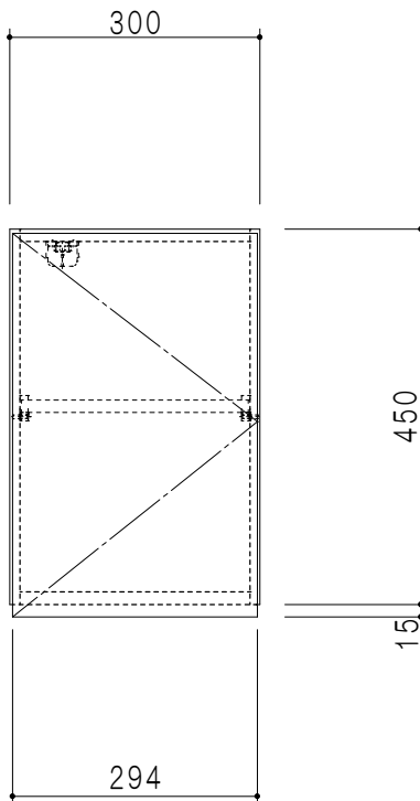
立面図
