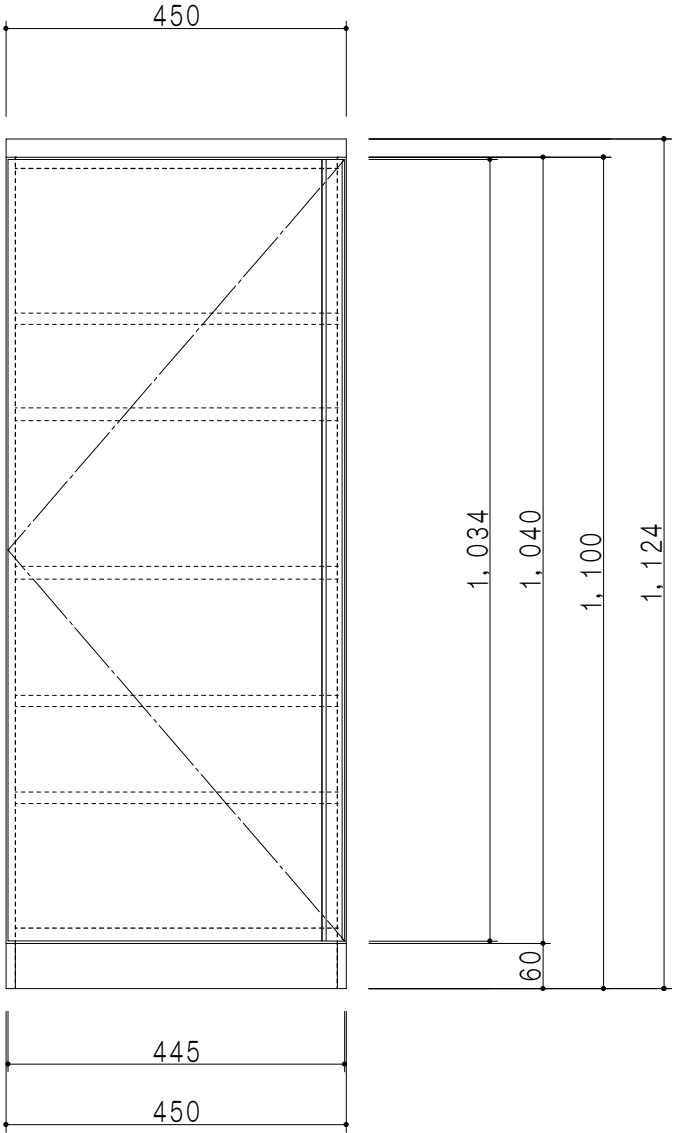
立面図
