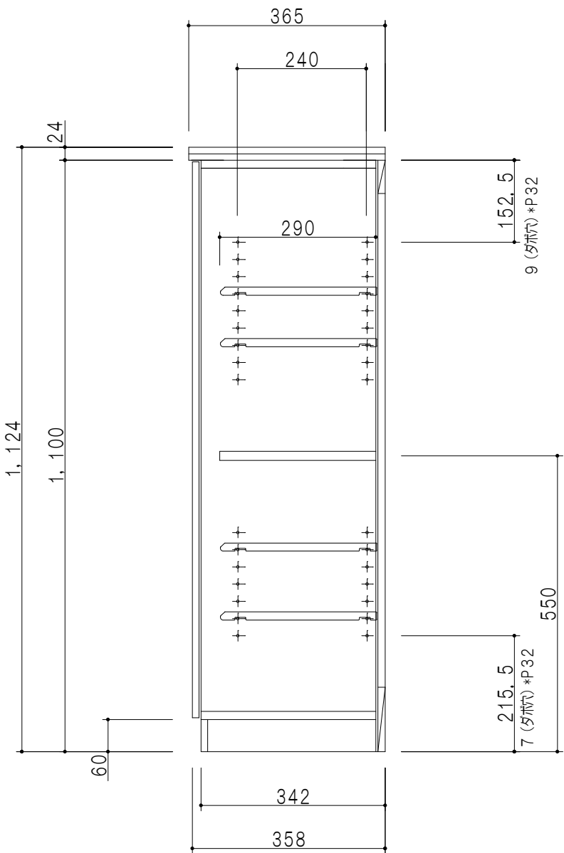
断面図
