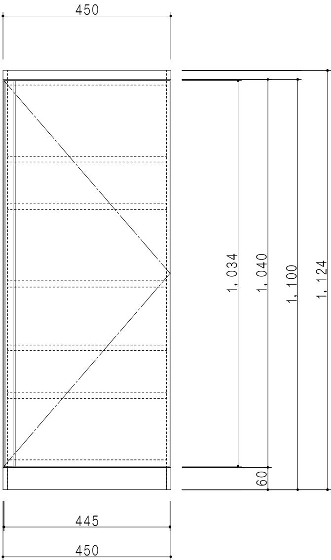
立面図
