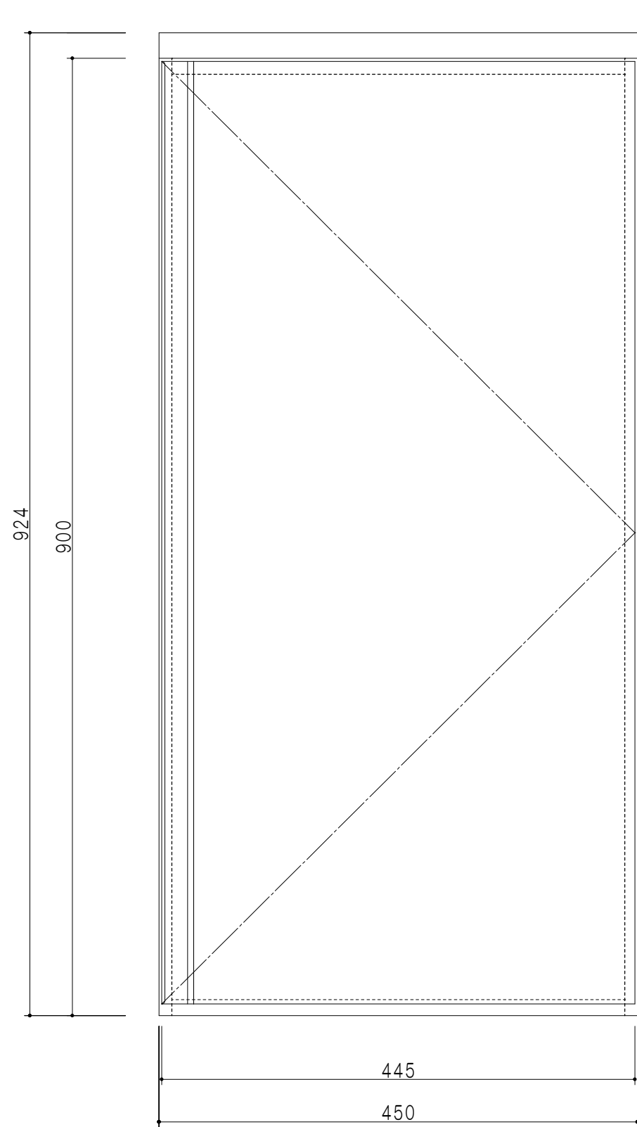
立面図
