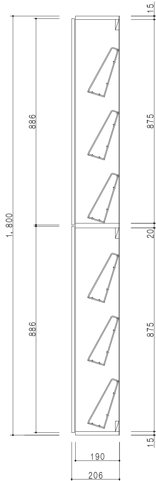
断面図
