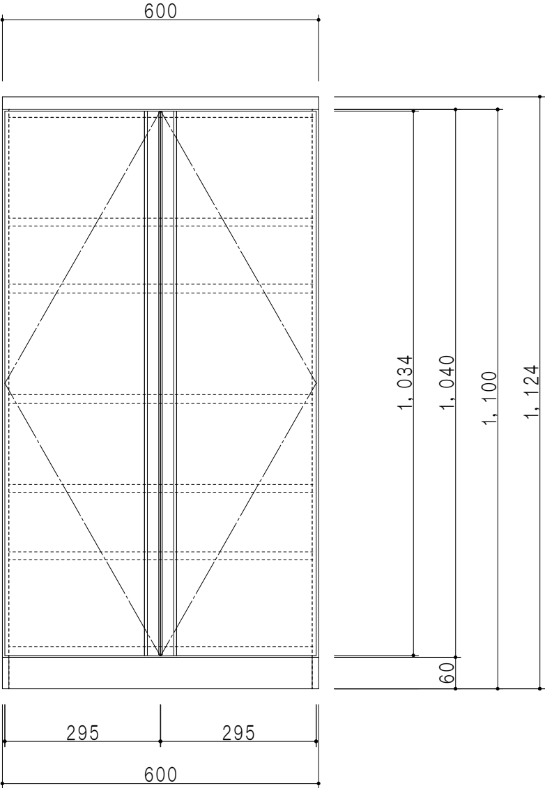
立面図
