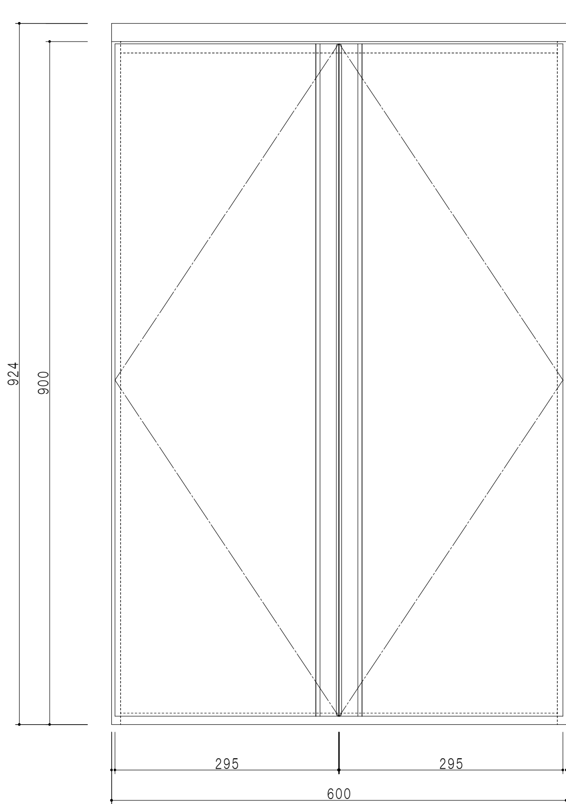
立面図
