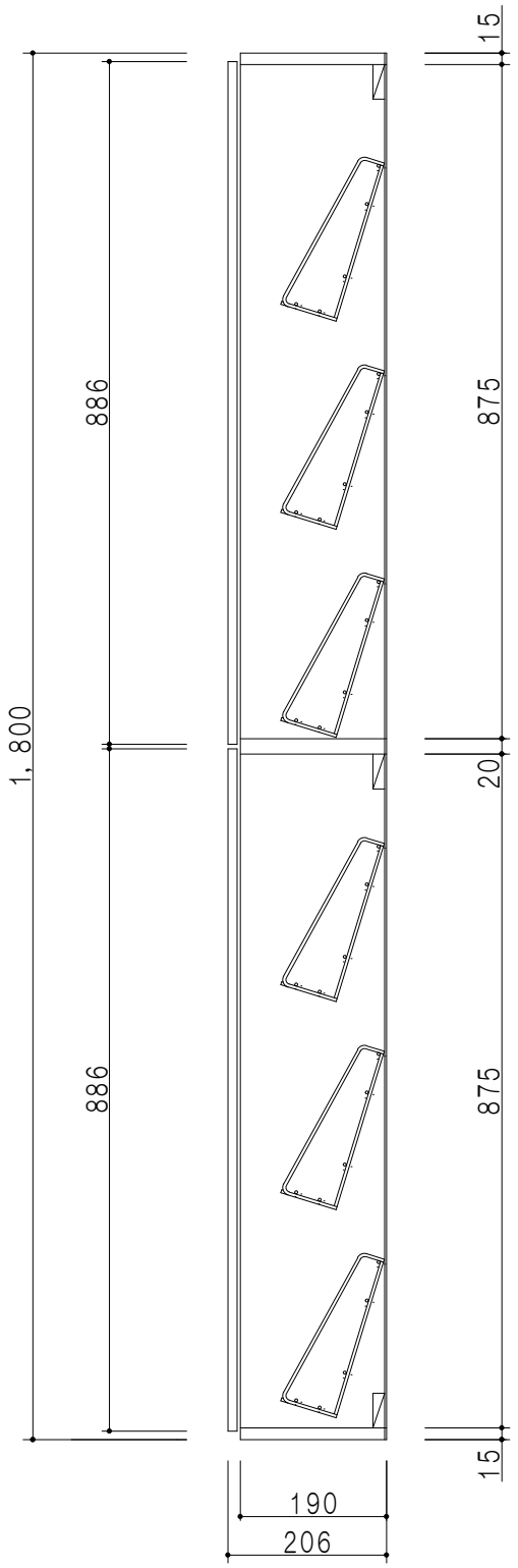
断面図
