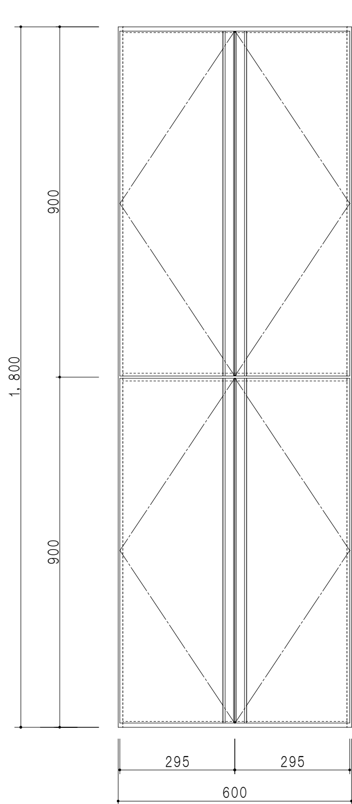
立面図
